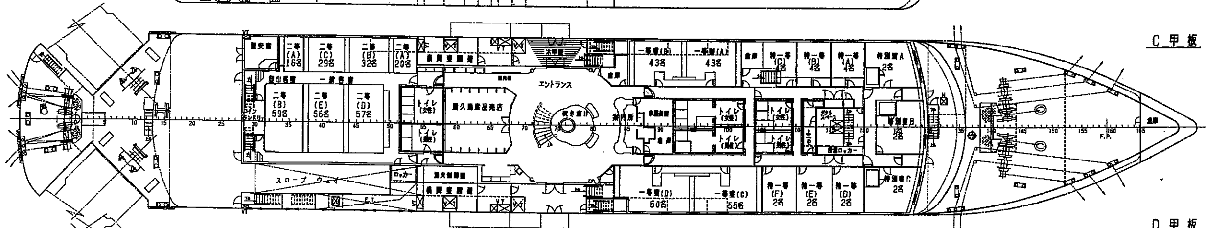
D甲板
