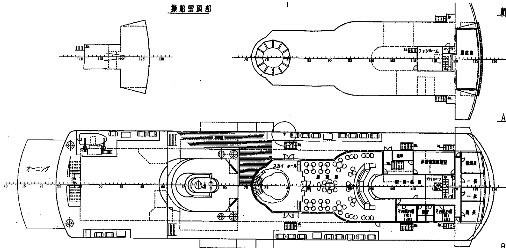
B甲板
