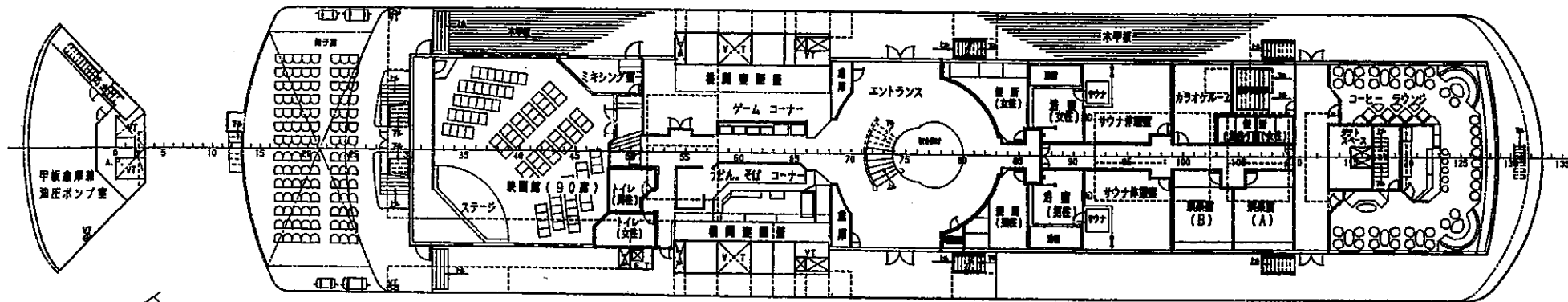
中間甲板
